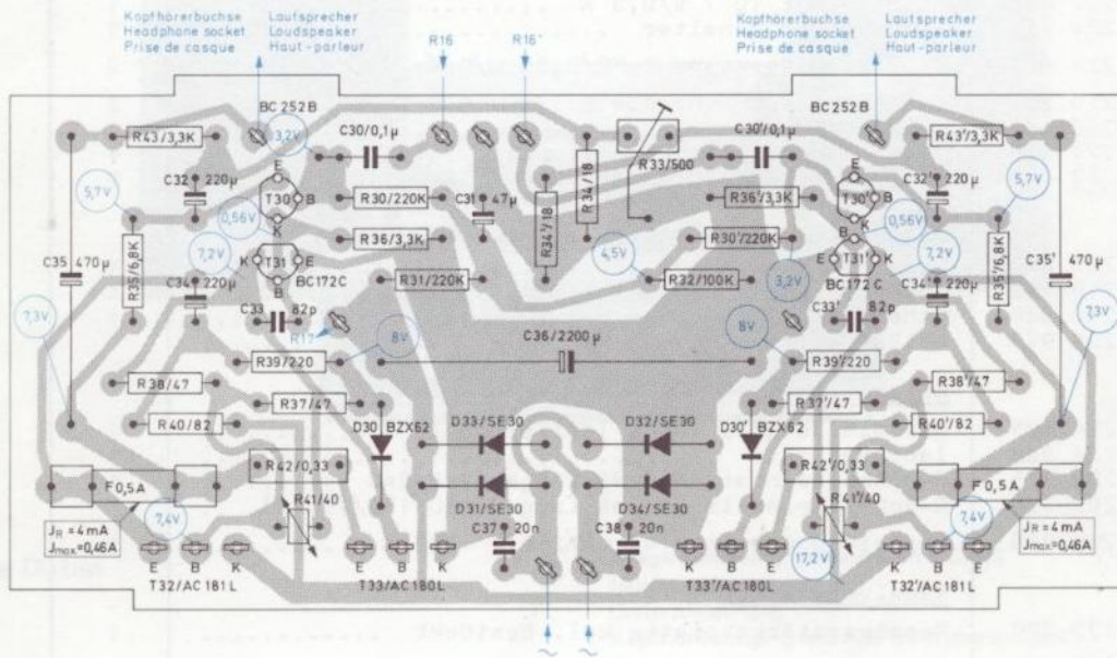
Fig. 3 Endverstärker 225 473 (Leiterseite)
